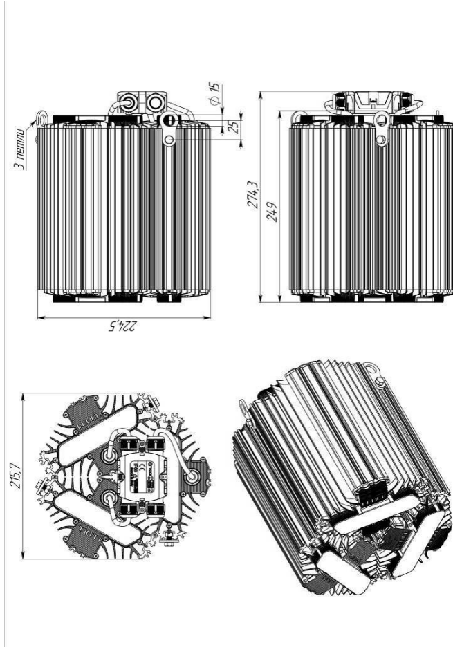
Рисунок 1 Светильник «L-lego 165». Подвесное крепление
