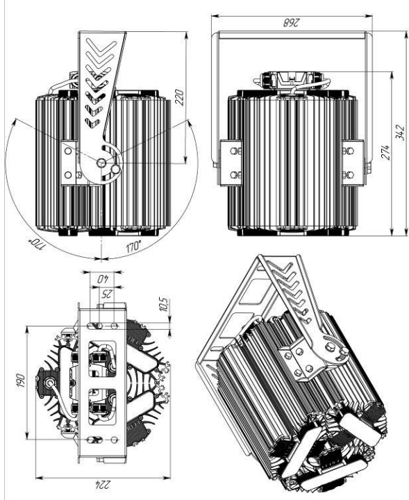
Рисунок 2 Светильник «L-lego 165 watt». Поворотное крепление.
