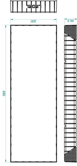
Рисунок 1а Светильники «L-school 16»
