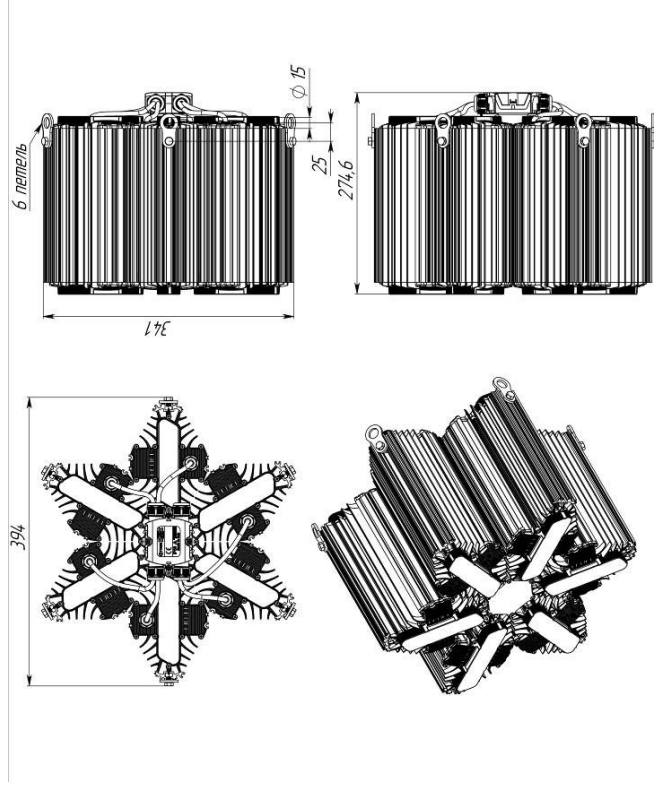
Рисунок 1 Светильник «L-lego 330». Подвесное крепление
