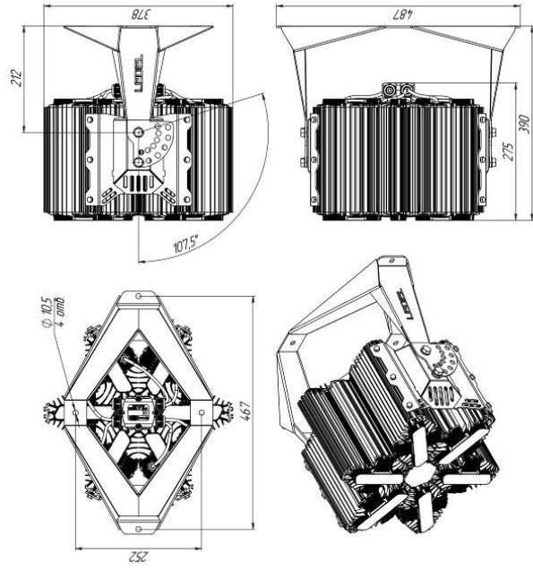
Рисунок 2 Светильник «L-lego 330 vanner» Поворотное крепление
